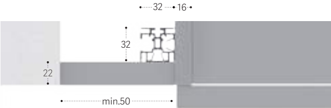
Tamponamento a filo fianco. Flush side panel.
