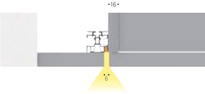
Tamponamento a filo anta, con luce diretta . Flush door panel with direct lighting.
